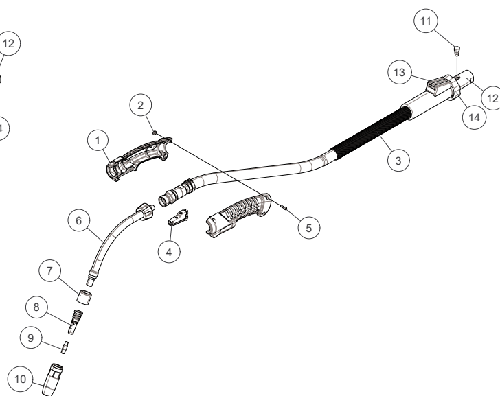
550A HDE Gun
